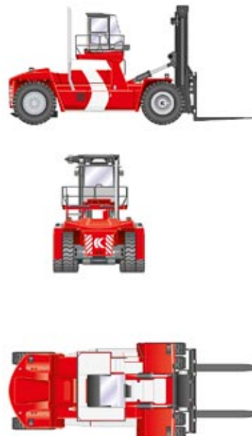
DCF450-12CS
